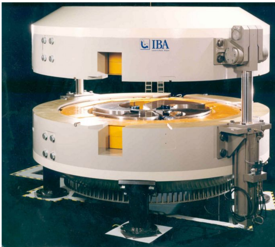
Рис. 1. Протонный циклотрон С235 – внешний вид
