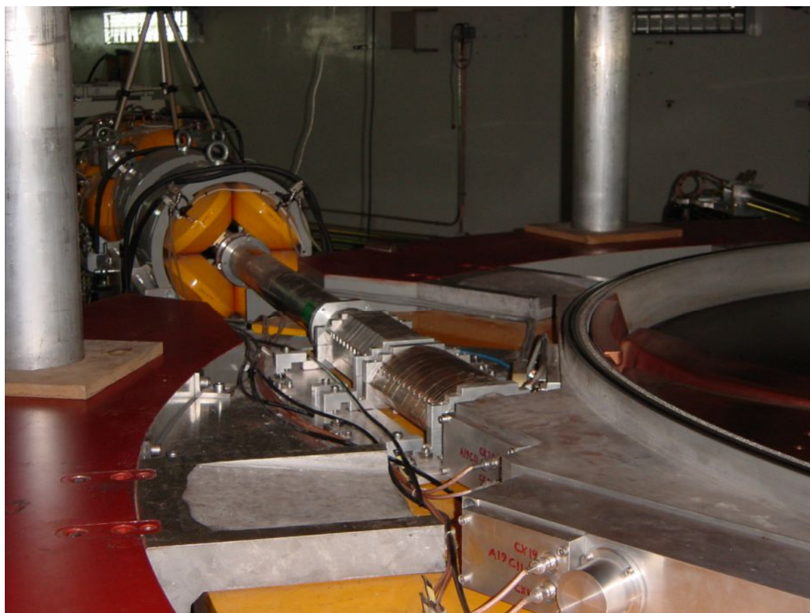
Рис. 7. Линия транспортировки пучка из циклотрона С235
