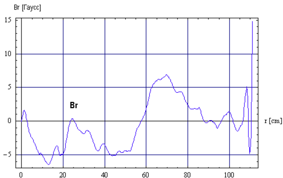
Рис. 3. Средняя (по азимуту) компонента- B_r в циклотроне С235 Р06
