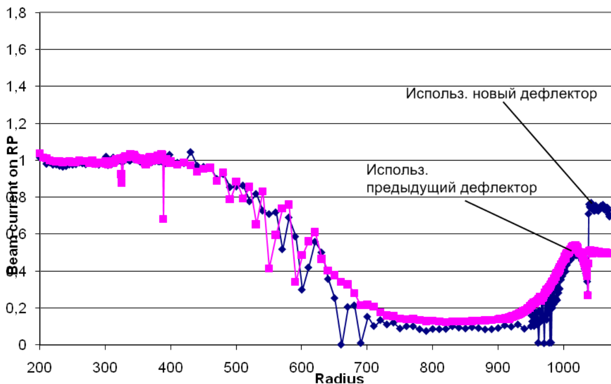
Рис. 9. Зависимость измеренной интенсивности тока пучка (нормирована на величину тока на радиусе 300мм) от радиуса в циклотроне С235 РАР-111 при использовании дефлекторов нового и предыдущего типов
