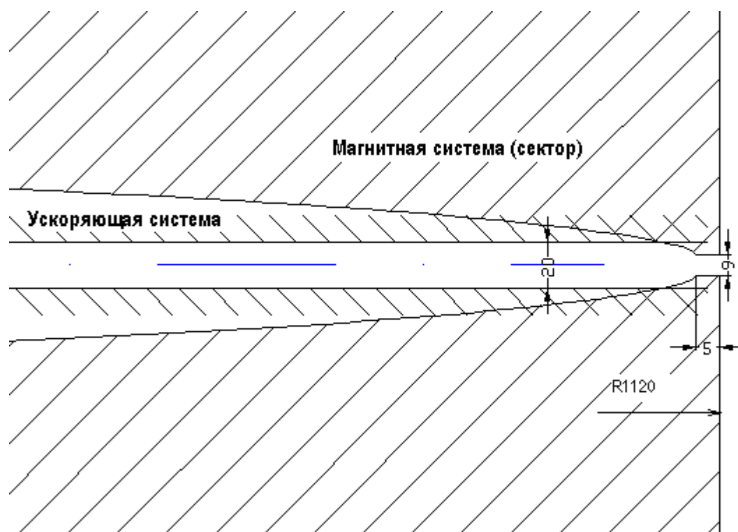
Рис. 4. Вертикальная апертура циклотрона С235
