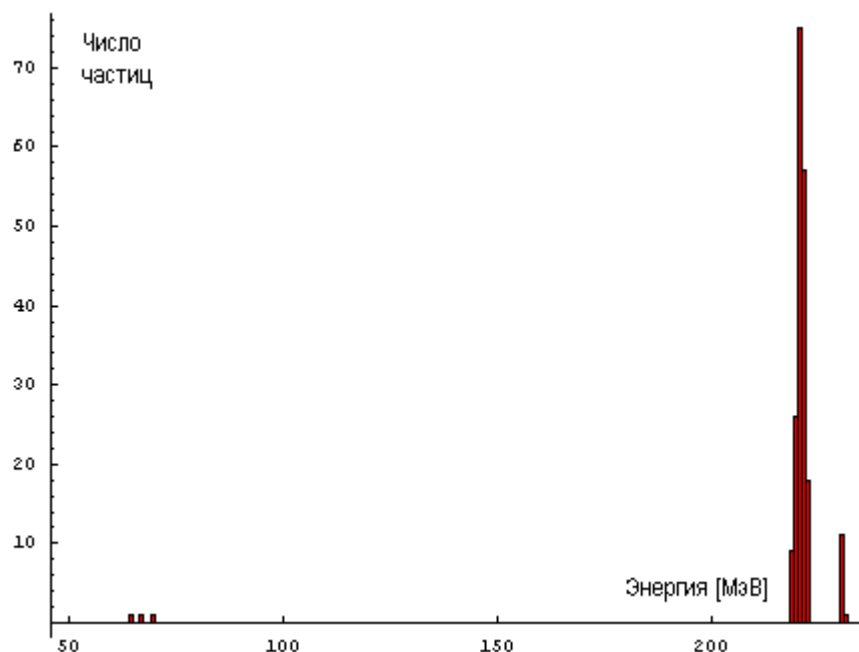
Рис. 6. Распределение потерянных частиц по энергиям
