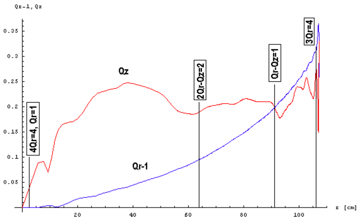
Рис. 2. Зависимость частот бетатронных колебаний от радиуса
