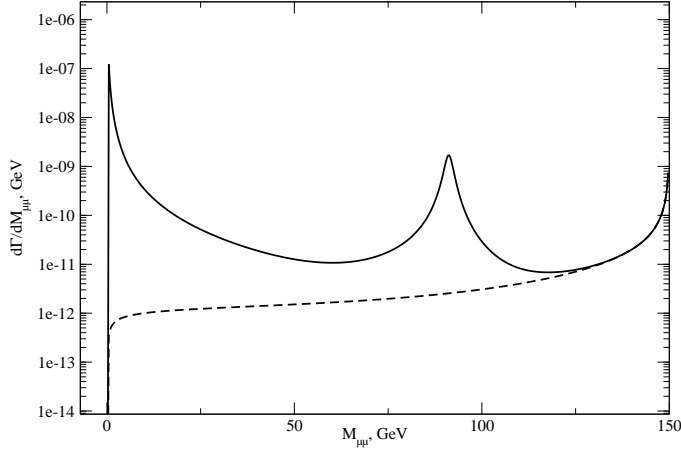
Рис. 2: Распределение по инвариантной массе \mu^+\mu^- пары. Показаны и борновский (пунктирная линия), и однопетлевой (сплошная) результаты.
