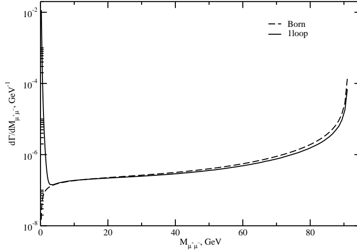
Рис. 3: Распределение по инвариантной массе \mu^+\mu^- пары распада Z \rightarrow \mu^+\mu^-\gamma(\gamma) . Представлены и борновский (пунктирная линия), и однопетлевой (сплошная линия) результаты.
