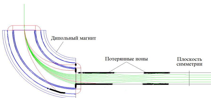
Рис. 12. Принцип работы системы отбора ионов.
