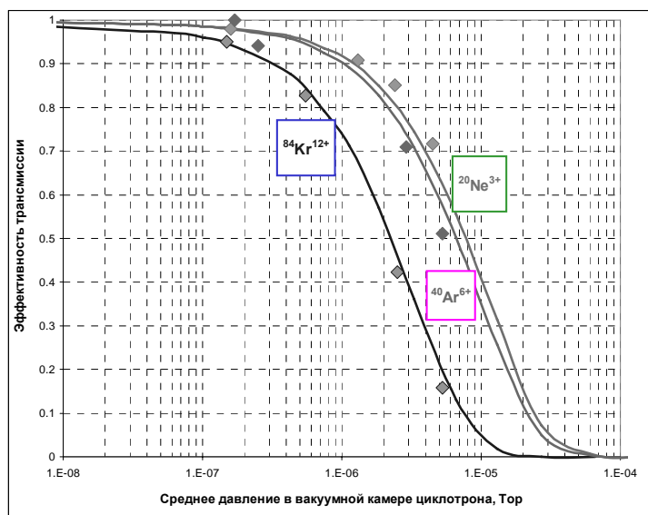
Рис. 7. Эффективности прохождения ускоренных пучков от центра до радиуса вывода R_{\text{выв}} = 68 см в вакуумной камере циклотрона DC-60 в зависимости от среднего давления в вакуумной камере циклотрона. Сравнение результатов моделирования и эксперимента по ускорению пучков ионов (символы – экспериментальные данные).
