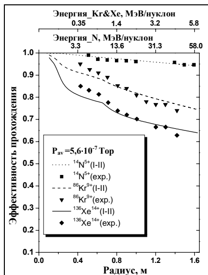
Рис. 5. Эффективности прохождения ускоряемых пучков в зависимости от радиусов орбит (и, соответственно, энергий – по верхней оси координат) в вакуумных камерах циклотронов У-400 для ионов ^{86}\text{Kr}^{9+} и ^{136}\text{Xe}^{14+} и У-400М для ионов ^{14}\text{N}^{5+} , символы – экспериментальные данные.
