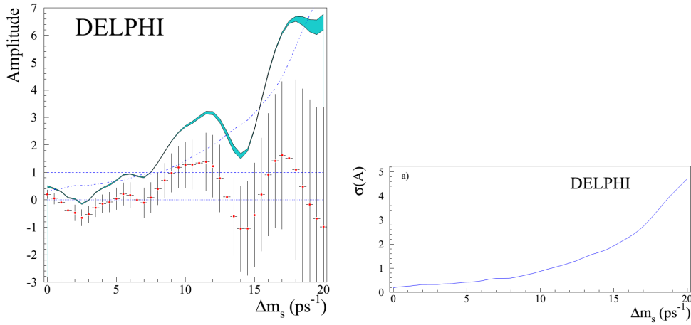
Рис. 5: (Слева) Изменение амплитуды осцилляций A в зависимости от \Delta m_{B_s^0} ( \Delta m_{B_s^0} \equiv \Delta m_s ). Точками с ошибками представлены экспериментальные данные. Цветная область, с изменяющимся контуром, соответствует зависимости амплитуды A + 1,645\sigma(A) с учётом систематических ошибок. Штрих-пунктирная линия соответствует кривой чувствительности. Также показаны линии A=0 и A=1 . (Справа) Зависимость ошибки в амплитуде \sigma(A) в зависимости от \Delta m_{B_s^0} , включая систематические неопределённости.
