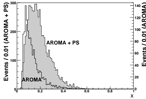
Рис. 25: Распределения долей импульса нуклона x , переносимых взаимодействующими глюонами, для D_{K\pi}^* событий Монте-Карло в ЛП КХД (помечено 'AROMA') и в ЛП КХД с партонным ливнем (AROMA + PS). Следует отметить различную нормировку распределений.
