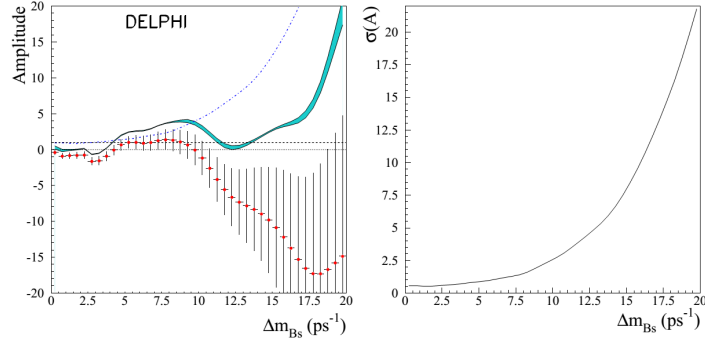
Рис. 8: (Слева) Изменение амплитуды осцилляций A в зависимости от \Delta m_{B_s^0} . Точки с ошибками представлены экспериментальные данные. Цветная область, с изменяющимся контуром, соответствует зависимости амплитуды A + 1,645\sigma(A) с учётом систематических ошибок. Штрих-пунктирная линия соответствует кривой чувствительности. (Справа) Зависимость ошибки в амплитуде \sigma(A) в зависимости от \Delta m_{B_s^0} , включая систематические неопределённости.
