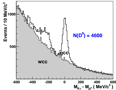
Рис. 20: Распределения инвариантной массы K\pi пары из выборки D_{K\pi}^* с правильной ( gcc ) и неправильной ( wcc ) комбинацией знаков заряда частиц. Использованы данные 2007 года, полученные на протонной ( NH_3 ) мишени.
