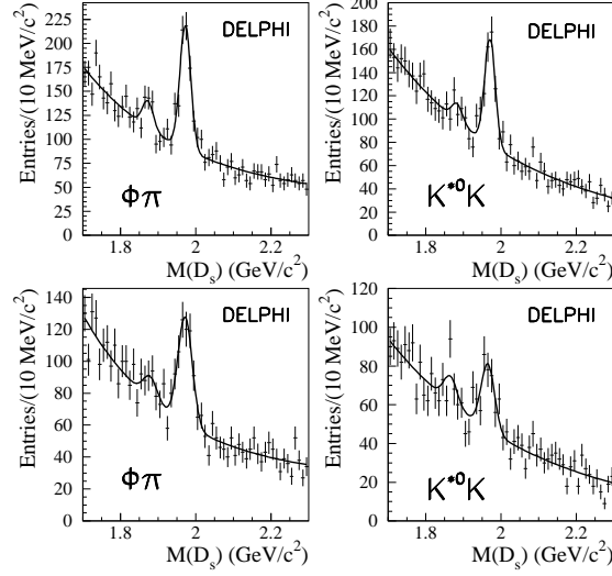
Рис. 6: Распределения инвариантных масс кандидатов в D_s мезоны, реконструированных в модах распада \phi\pi^- и K^{*0}K^- , после выбора адрона сопровождения. Верхний ряд соответствует 1994-1995 гг., а нижний 1992-1993 гг. набора данных.
