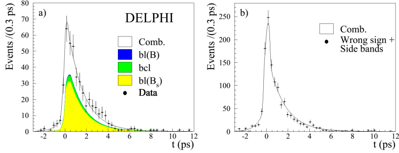
Рис. 3: а) Фит методом правдоподобия распределения времён распада B_s^0 кандидатов из области сигнала [1,94 - 2,00] ГэВ/ c^2 (рис. 2-а) D_s^\pm 1^\mp выборки. Точками показаны данные, а кривые соответствуют вкладам различных компонент, оцененных методом Монте-Карло. б) Такое же распределение, как и а), но для событий с "неправильным" знаком и событий, лежащих вне области сигнала [1,91 - 1,93] & [2,01 - 2,15] ГэВ/ c^2 .
