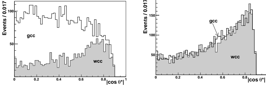
Рис. 21: Распределения |\cos \theta^*| (полярного угла К мезона в системе центра масс D^0 мезона по отношению к импульсу D^0 ) в лабораторной системе D^0 мезона для g_{cc} и w_{cc} событий ( D_{K\pi}^* выборка данных 2006 года). Слева события из зоны сигнала (в пределах \pm 40 МэВ/ c^2 от номинальной массы D^0 мезона), справа события из зоны вне сигнала.
