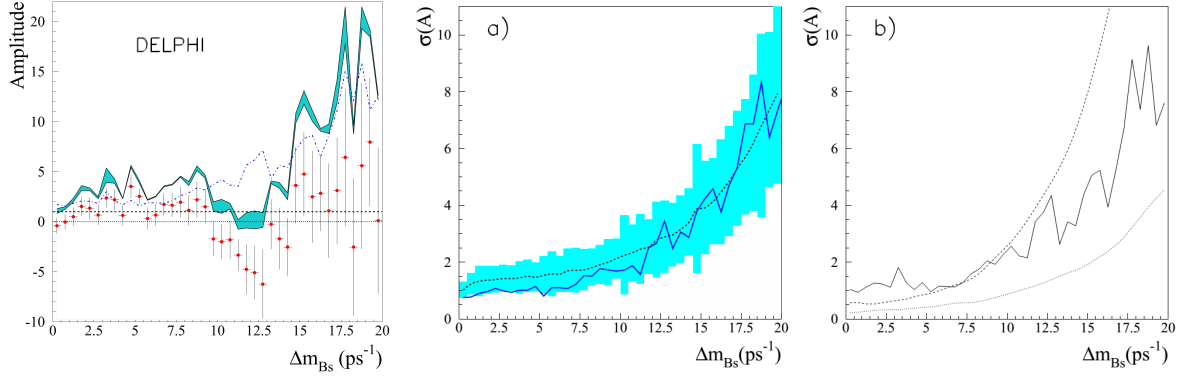
Рис. 11: (Слева): Изменение амплитуды осцилляций A в зависимости от \Delta m_{B_s^0} . Точками с ошибками представлены экспериментальные данные. Цветная область, с изменяющимся контуром, соответствует зависимости амплитуды A + 1,645\sigma(A) с учётом систематических ошибок. Штрих-пунктирная линия относится к кривой чувствительности. а): Сплошная линия показывает изменение ошибки амплитуды осцилляций \sigma(A) в зависимости от \Delta m_{B_s^0} . Пунктирная линия показывает изменение усреднённой ошибки \sigma(A) , полученной на 100 Монте-Карло выборках B_s^0 мезонов со статистикой эквивалентной статистике экспериментальных данных. Цветом показана область \pm 2\sigma(A) вокруг среднего без учёта систематических ошибок. б): Сравнение ошибок \sigma(A) в зависимости от \Delta m_{B_s^0} для трёх анализов: сплошная линия соответствует эксклюзивному B_s^0 анализу, а штриховая и пунктирные линии показывают результаты D_s^\pm h^\mp и D_s^\pm l^\mp анализов соответственно.
