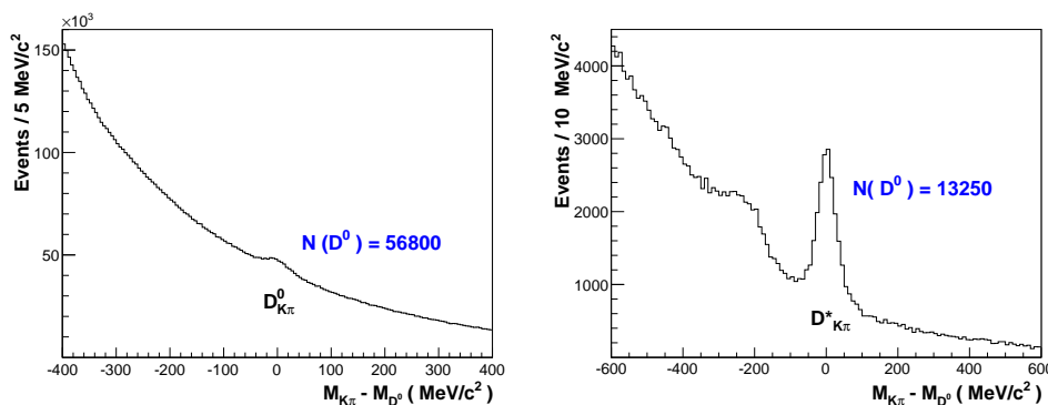
Рис. 18: Спектры инвариантных масс D_{K\pi}^0 (слева, "немеченая" выборка) и D_{K\pi}^* (справа, "меченая" выборка) кандидатов. Указано приблизительное число D^0 мезонов в пиках.
