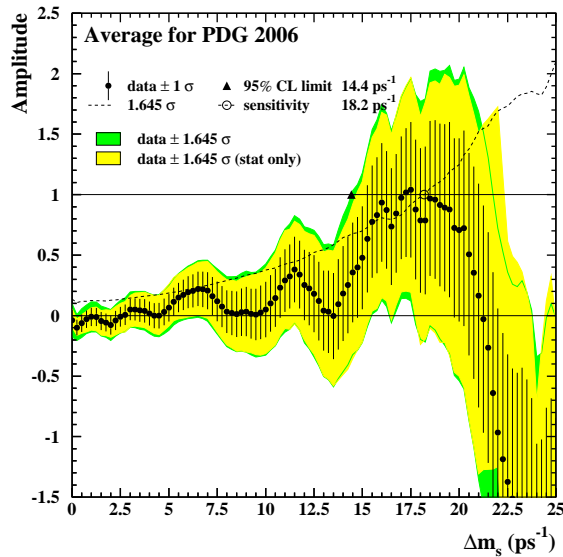
Рис. 13: Значения амплитуды A осцилляций B_s^0-\bar{B}_s^0 в 2006 году до измерения \Delta m_{B_s^0} на CDF. Верхний рисунок: вклады отдельных экспериментов с указанием использованного метода измерения \Delta m_{B_s^0} . Нижний рисунок: зависимость амплитуды осцилляций A от \Delta m_{B_s^0} . Точками с ошибками показаны экспериментальные данные. Пунктирная линия представляет кривую чувствительности. На рисунках \Delta m_s \equiv \Delta m_{B_s^0} .
