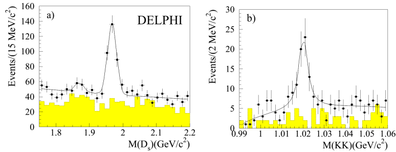
Рис. 2: Распределения инвариантных масс а) D_s кандидатов с адронными модами распада \phi\pi^- , K^{*0}K^- , K_S^0K^- , K^{*0}K^{*-} , \phi\pi^-\pi^+\pi^- и \phi\pi^-\pi^0 ; б) K^+K^- мезонов от распадов \phi кандидатов, отобранных в двух полулептонных модах распада D_s ( \phi\mu^-\nu_\mu и \phi e^-\nu_e ). Соответствующие распределения инвариантных масс для событий с "неправильным" знаком показаны в виде гистограмм.
