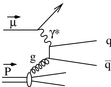
Рис. 15: Диаграмма ФГС, используемая для прямого измерения поляризации глюонов \Delta g/g в мюонном пучке.
