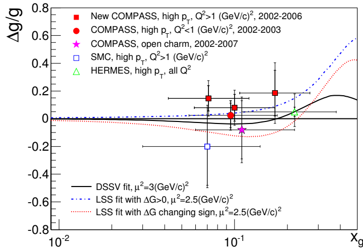
Рис. 23: Мировые результаты прямых измерений поляризации глюонов в ЛП КХД, выполненные методом "открытого очарования" и методом "больших p_T ". Горизонтальная черта указывает на интервал по x_g ( x_g \equiv x ) каждого измерения, а вертикальная на статистическую неопределённость или полную точность.
