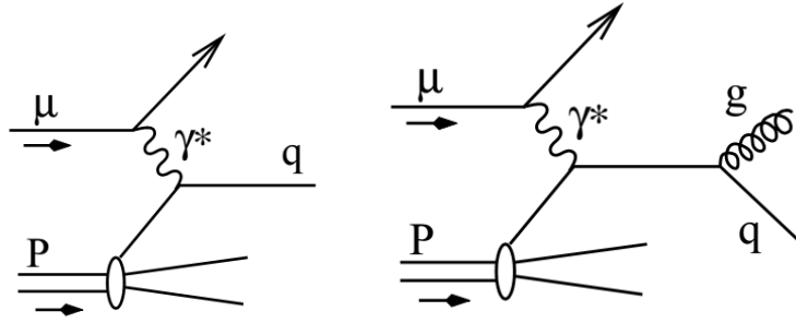
Рис. 16: Диаграммы фоновых процессов к реакции ФГС при измерении \Delta g/g методом "больших p_T ": слева реакция ГНР в ЛП КХД, а справа комптоновское КХД рассеяние.
