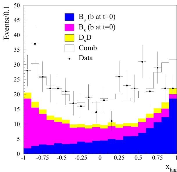
Рис. 4: Распределение переменной маркировки x_{tag} для D_s^{\pm 1\mp} выборки. Точками с ошибками представлены экспериментальные данные. Цветные гистограммы получены методом Монте-Карло. Белая гистограмма представляет комбинаторный фон, жёлтая гистограмма вклад от D_s D событий, более тёмные гистограммы показывают вклады от \bar{B}_s^0 мезонов с b -кварком и B_s^0 мезонов с \bar{b} -кварком.
