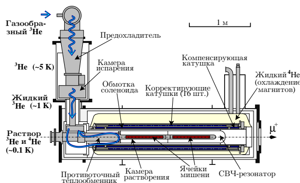
Рис. 17: Схематический вид сбоку на поляризованную мишень COMPASS. Стрелками показан маршрут циркуляции хладагента ^3\text{He} внутри мишени. Основные компоненты системы: криогенное оборудование, сверхпроводящий магнит, два многомодовых СВЧ-резонатора и приспособление для измерения поляризации (Q-метр)
