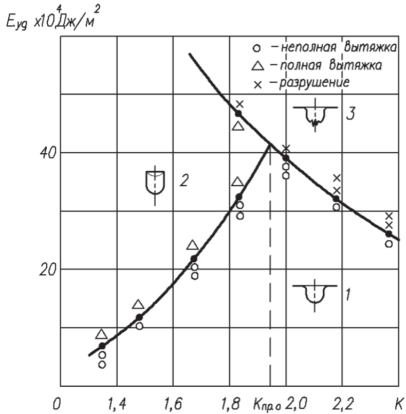
Рисунок 1: Диаграмма штампуемости сверхчистого ниобия
