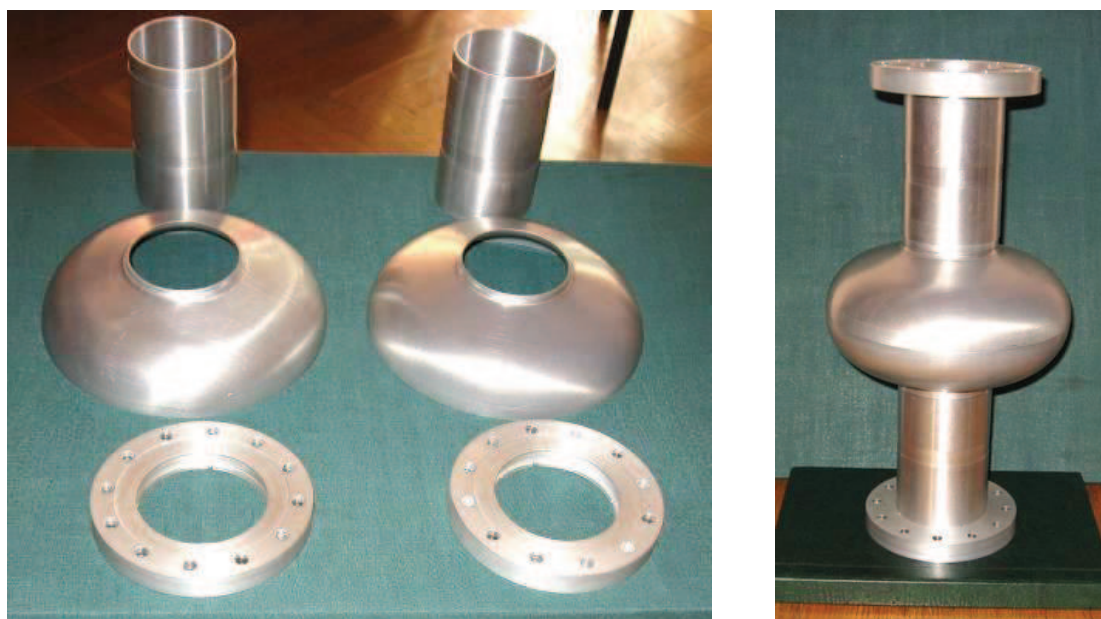
Рисунок 2: Изготовленные детали одноячеечного резонатора из ниобия (слева) и резонатор в сборе (справа)
