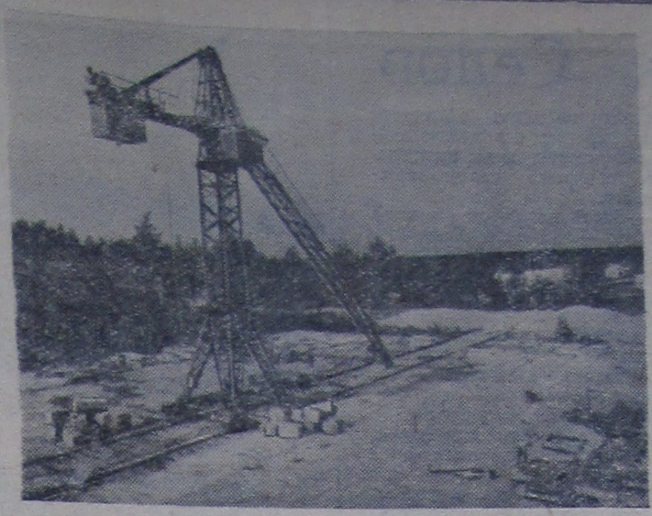
На заводе железобетонных изделий работает открытый полигон, который дает стройкам Дубны сотни кубометров сборного бетона. Большинство работ здесь механизировано. На снимке: монтаж башенного крана на открытом полигоне. Фото П. Зольникова.
