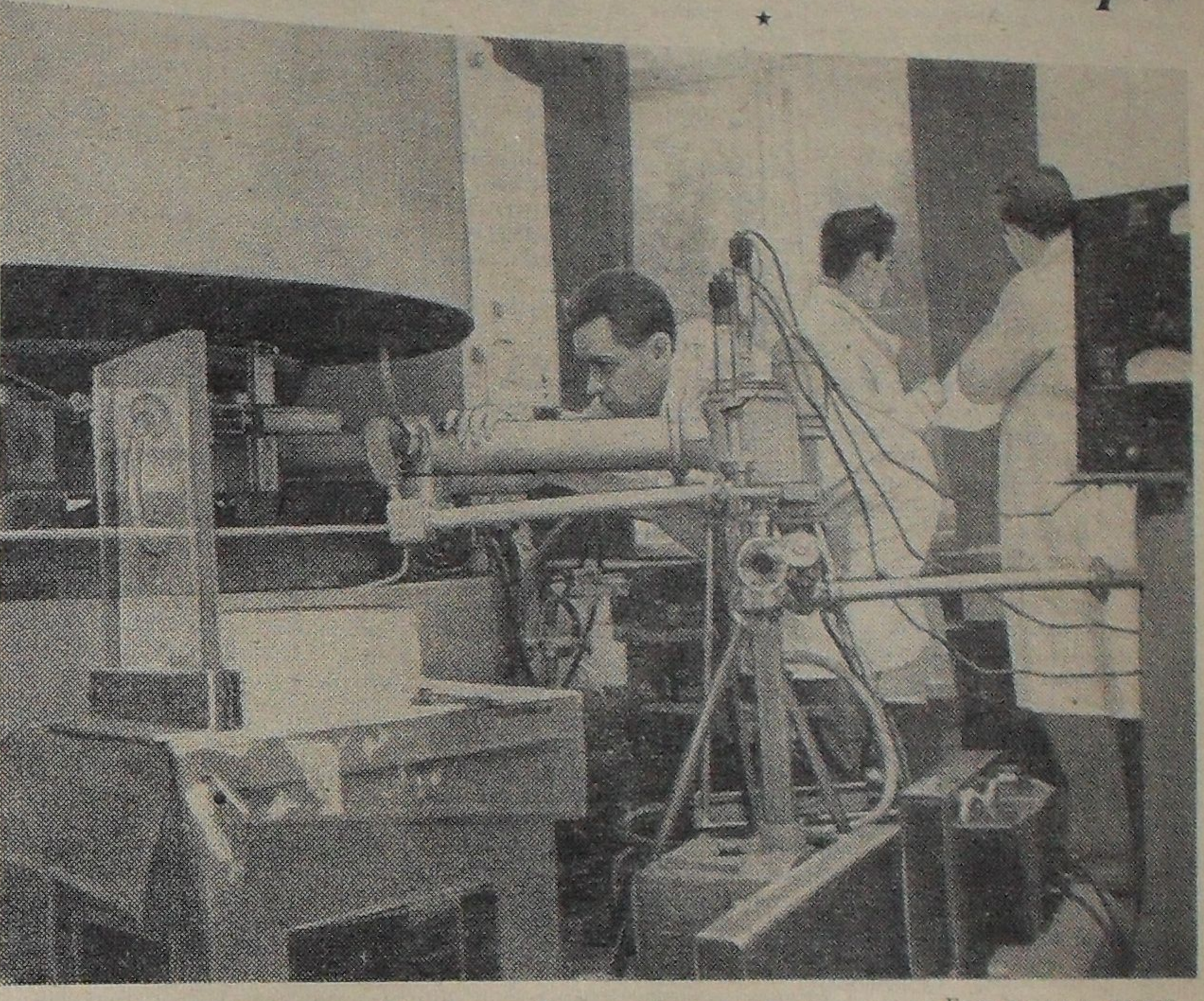
Этот прибор называется бета-спектрометр с двухкратной двойной фокусировкой электронов. На нем ведутся измерения спектров конверсионных электронов изотопов редкоземельной области. Прибор работает с очень малым фоном, что позволяет наблюдать эффекты очень малой интенсивности.
