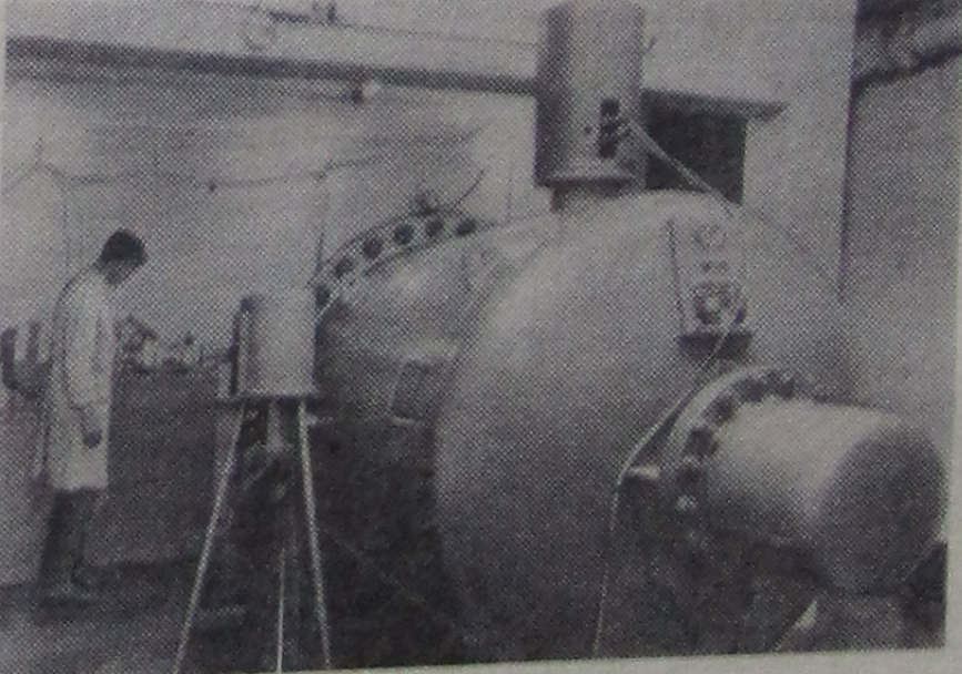
На снимке: электростатический генератор россендорфского научного центра.
