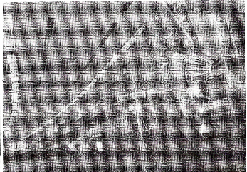
Установка, используемая в эксперименте по поиску тяжелых частиц и антиядер (отв. В. И. Петрухин), в настоящее время модернизирована и полностью готова к проведению завершающего этапа (предварительные результаты были получены в 1970 г.).
