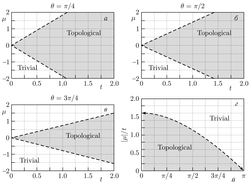
а–в) Зависимость тривиальной и топологической фазы от угла поворота спина через соседние узлы ( \theta ). г) Условие |\mu|/t < 2 \cos(\theta/2) , определяющее топологическую фазу
