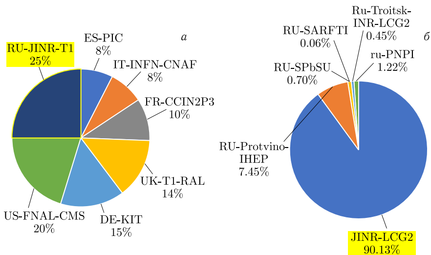
Распределение по нормированному времени загрузки CPU в HS23 часах за 2024 г. для Tier-1 сайтов для эксперимента CMS (а) и Tier-2 сайтов, входящих в консорциум RDIG (б)
