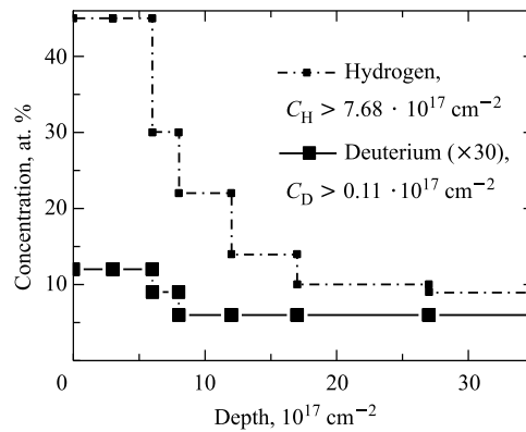
Рис. 8. Распределение водорода и дейтерия в приповерхностном слое 1 Nb-2-фольги
