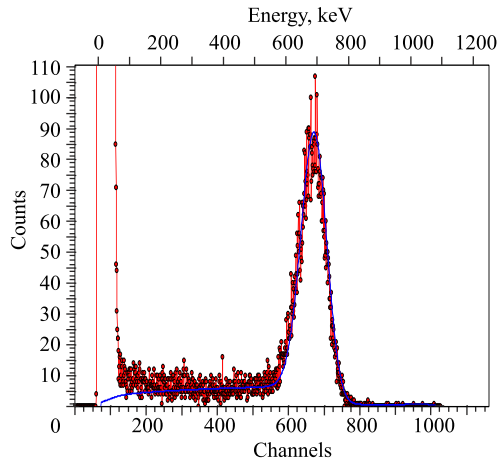
Рис. 2. Спектр упругорассеянных ядер отдачи водорода и дейтерия из приповерхностного слоя {}^1\text{Nb-1} -фольги
