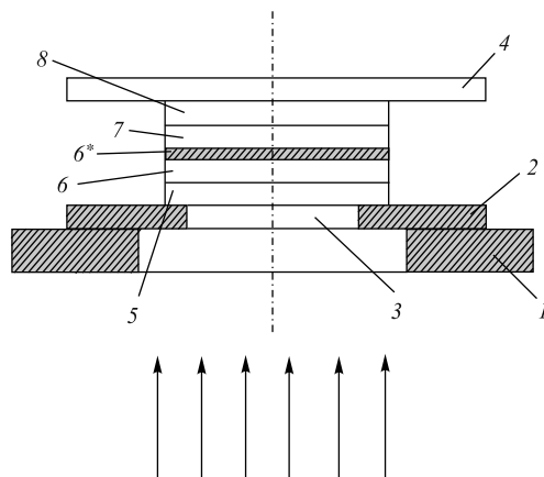
Рис. 1. Сборка Nb-фольг для изучения воздействия импульсов высокотемпературной плазмы на образцы на ПФ-4 [3, 7–9] (поток снизу). 1 — нижняя часть дискового держателя образцов на четыре сборки из нержавеющей стали X18H10T (НС); 2 — передняя диафрагма с диаметром отверстия 3, равным 10 или 15 мм; 4 — прижимная пластина из НС, а 5–8 — набор фольг из одного или различных материалов. Символ 6* означает, что фольга подвергнута с зачерненной стороны некоторой обработке
