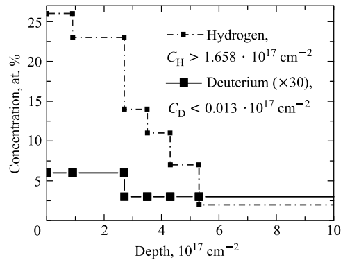
Рис. 3. Распределение водорода и дейтерия в приповерхностном слое {}^1\text{Nb-1} -фольги
