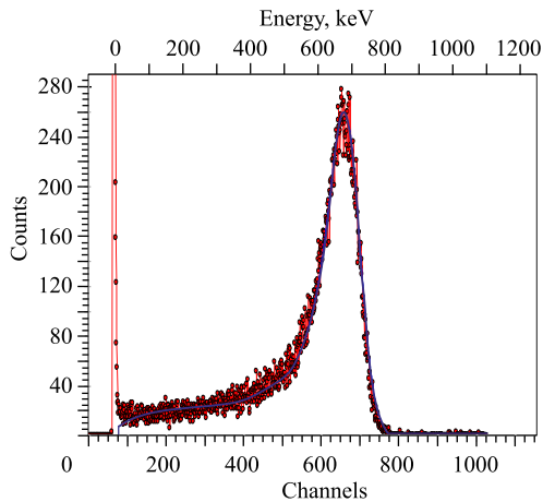
Рис. 7. Спектр упругорассеянных ядер отдачи водорода и дейтерия из приповерхностного слоя 1 Nb-2-фольги
