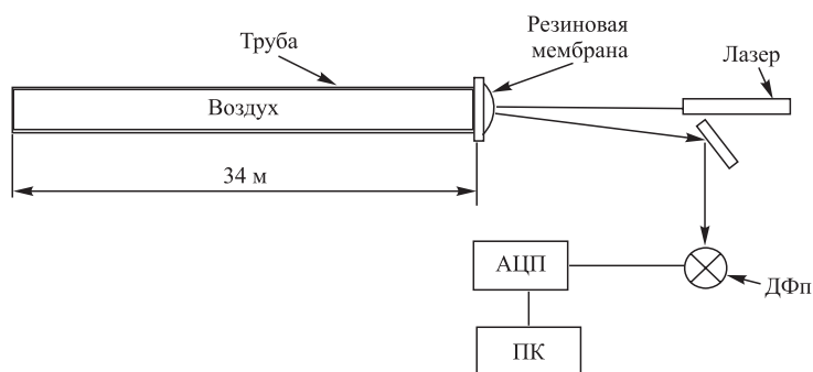
Рис. 5. Схема эксперимента с резиновой мембраной
