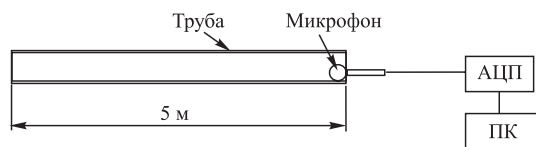
Рис. 8. Эксперимент с микрофоном на длине трубы 5 м
