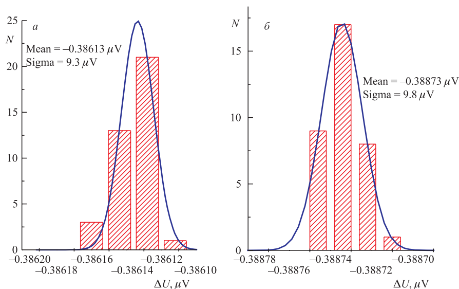
Рис. 3. Гистограммы, полученные из данных, соответствующих участкам А и Б на рис. 2
