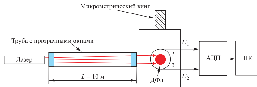
Рис. 1. Экспериментальная установка
