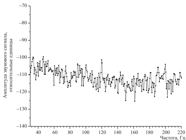
Рис. 12. Фурье-спектр звуковых колебаний воздуха вне трубы
