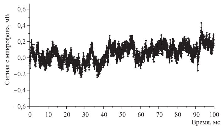
Рис. 11. Осциллограмма звуковых колебаний воздуха вне трубы
