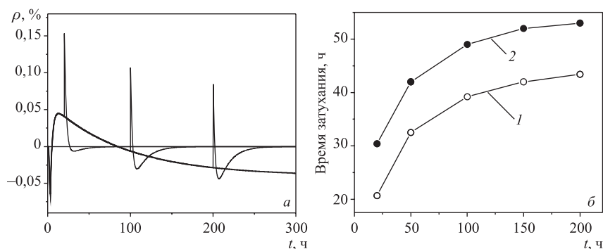
Рис. 2. Изменение реактивности обратной связи при единичном сбросе мощности в разные моменты времени от начала цикла (а) и время затухания эффекта сброса (б). 1 — погрешность 0,004 %; 2 — 0,002 %. Жирной линией показан ход мощностной обратной связи без сброса мощности
