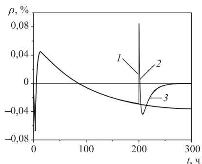
Рис. 1. Изменение реактивности обратнй связи в цикле при сбросе мощности в зависимости от времени: 1 — быстрая обратнй связь; 2 — действие медленной положительной компоненты обратнй связи; 3 — действие самого медленного звена обратнй связи. Жирной линией обозначен ход реактивности обратнй связи без сброса мощности
