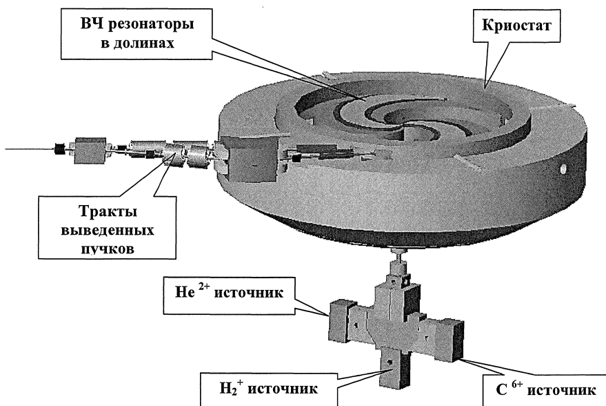
Рис. 1. Общий вид циклотрона С400
