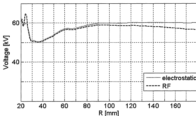
Рис. 4. Зависимость напряжения ускоряющего поля от радиуса
