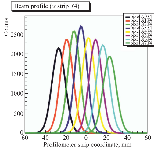
Рис. 3. Пространственные распределения нейтронов в меченых пучках
