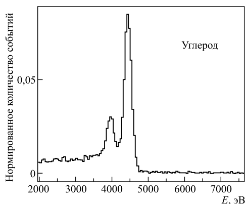
Рис. 4. Энергетический спектр гамма-квантов для графита (углерода)
