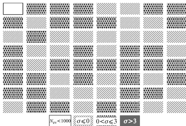
Рис. 7. Распределение \Delta_i = N - N_i для образца кимберлита №3
